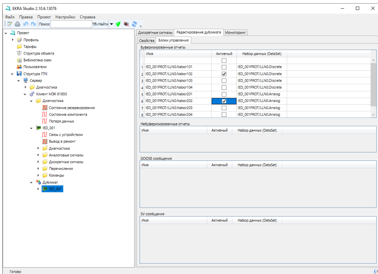
Рисунок 37 – Редактирование свойств дублируемого устройства клиента МЭК 61850
