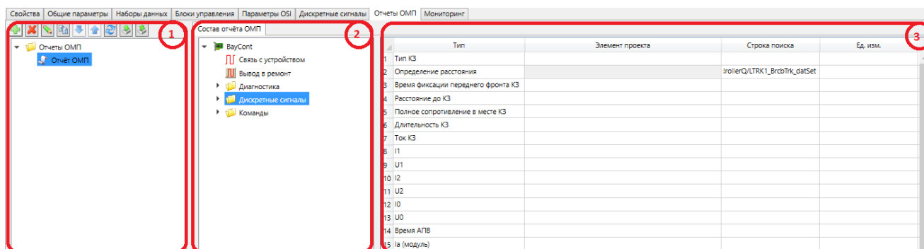
Рисунок 27 – Раздел «Отчеты ОМП»
