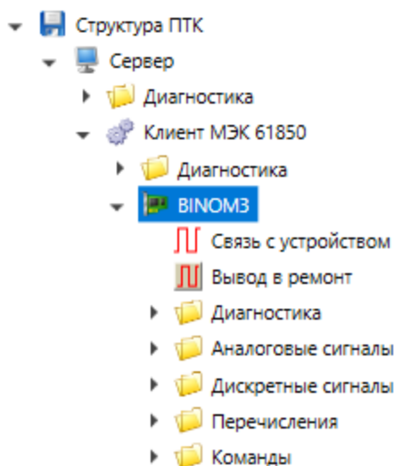
Рисунок 8 – Добавление устройства из файла конфигурации завершено
