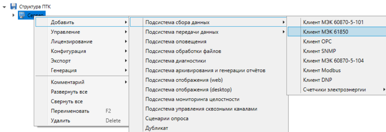
Рисунок 1 – Добавление компонентов подсистемы сбора данных
