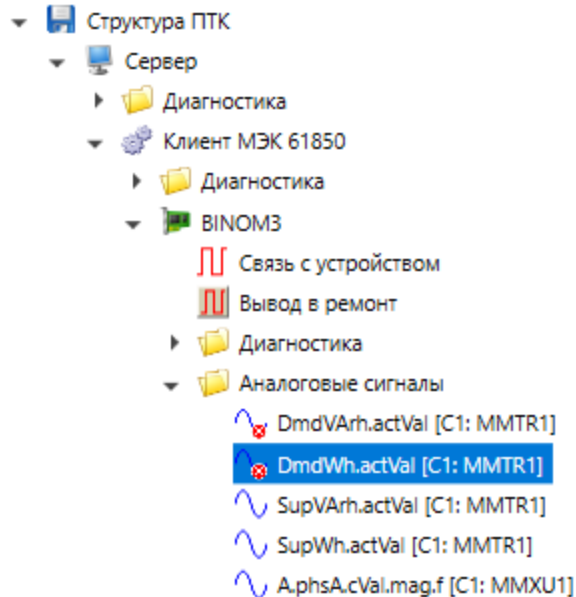
Рисунок 33 – Вид сигнала отключенного от опроса
