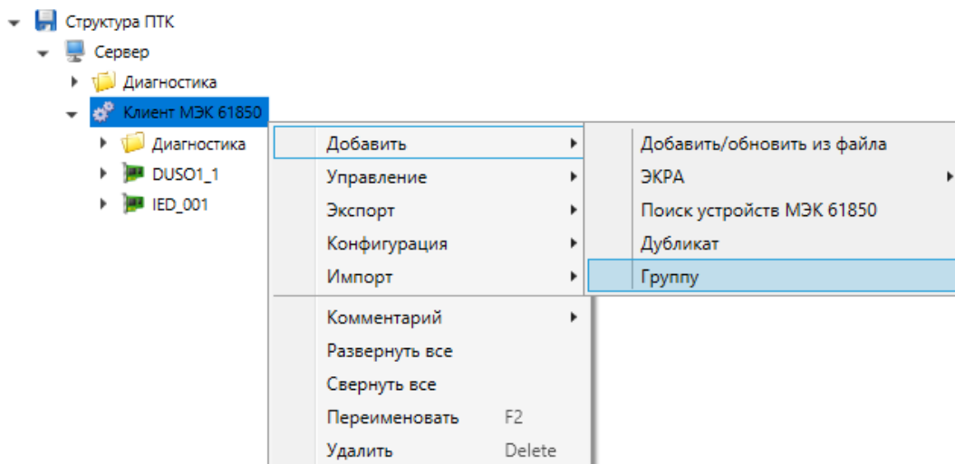
Рисунок 12 – Добавление группы
