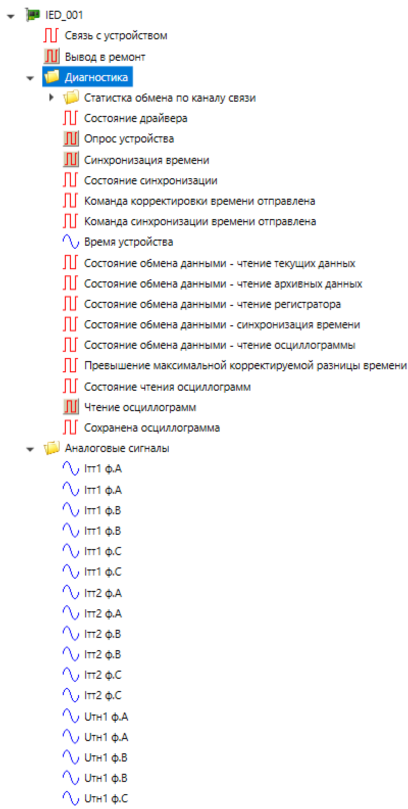
Рисунок 20 – Структура устройства МЭК 61850
