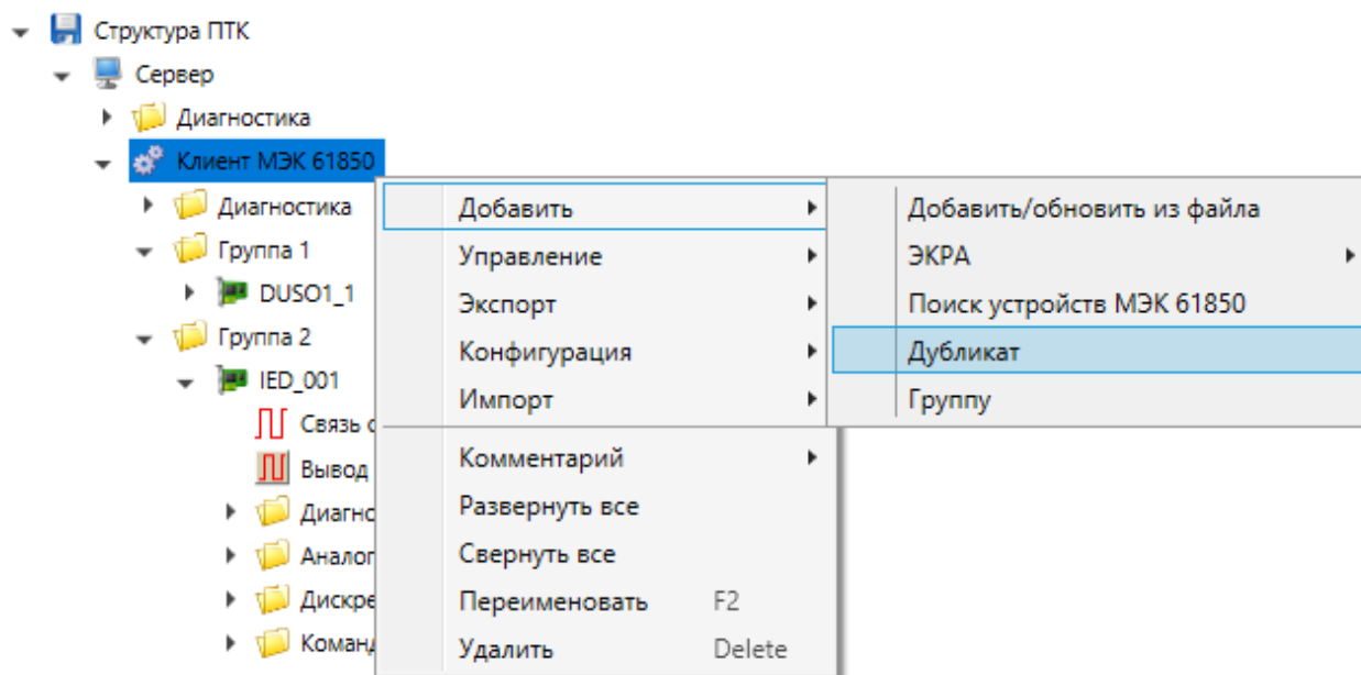
Рисунок 34 – Добавление дубликата
