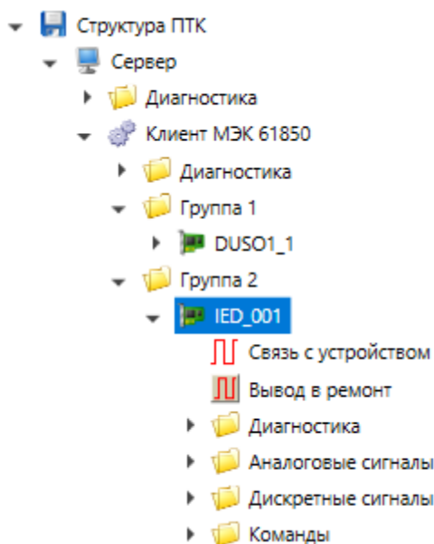
Рисунок 13 – Группировка устройств
