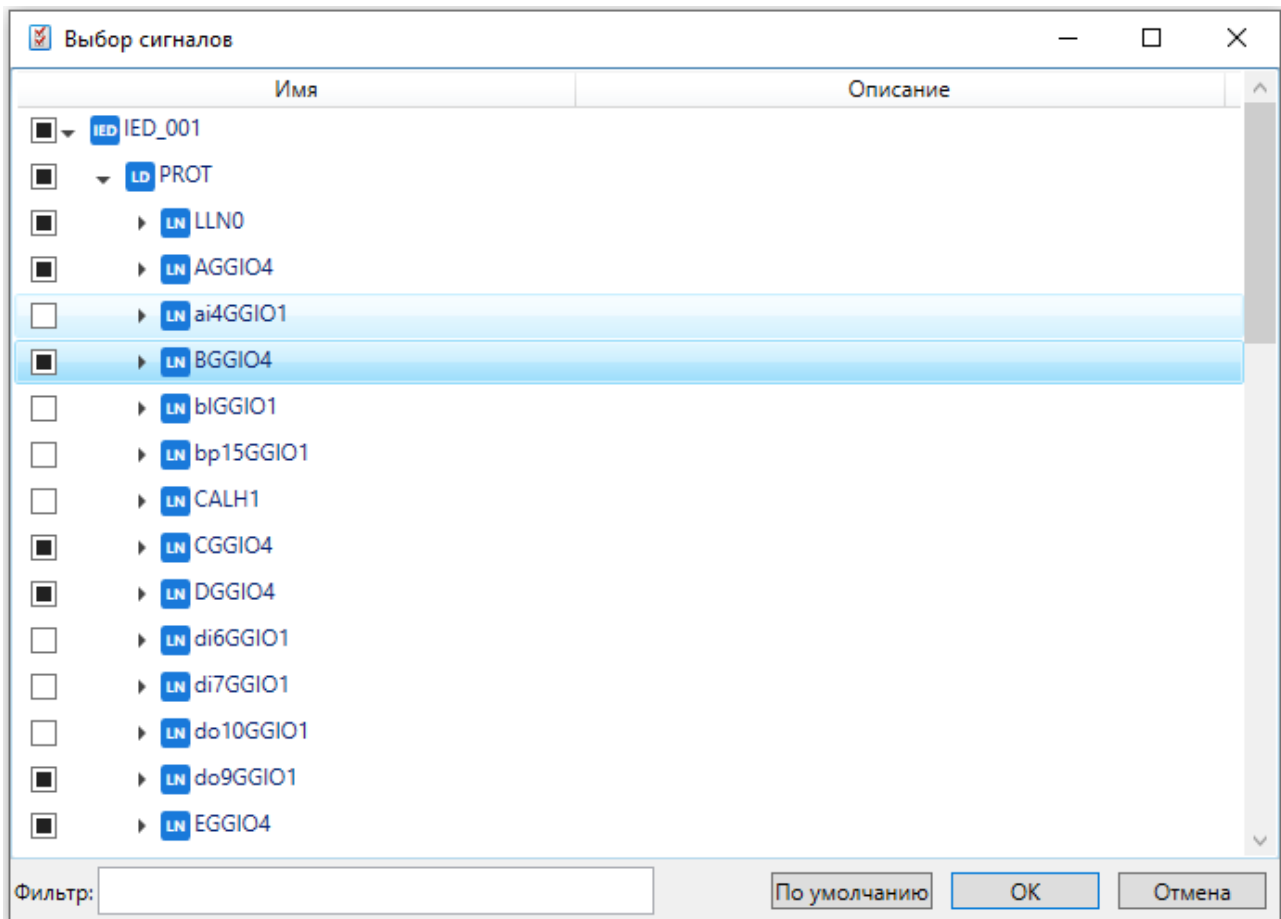
Рисунок 22 – Выбор сигналов
